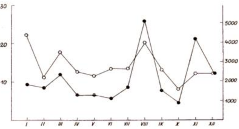
Rys. 1. Zmiany średniej miesięcznej powierzchni plam (kółka) i średniej miesięcznej promieniowania radiowego 127 Mc/s (kropki)
