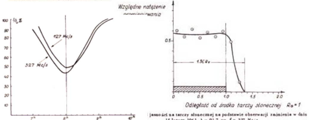
Rys. 1. Krzywe zaćmienia Słońca w dniu 15 lutego 1961 roku
